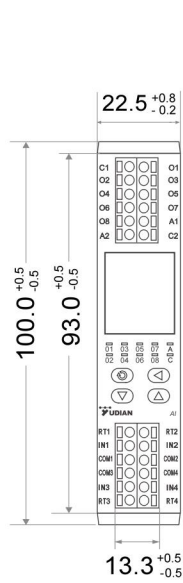
主视图
